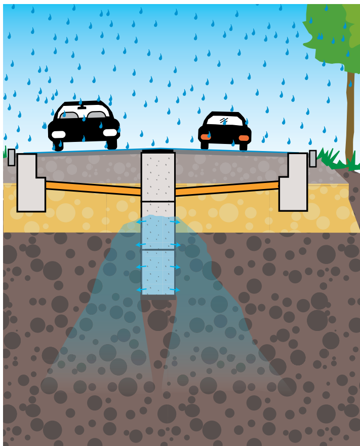
Regnvand ledes fra vejbrønde til IBF Perma-brønd for nedsvivning.
